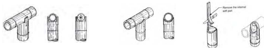
Gambar 2. Contoh Sambungan Bambu Sumber: Dunkelberg, Klaus (1985). IL 31 Bamboo.
