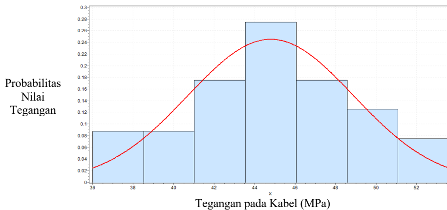
Gambar 10. Distribusi Fungsi Tegangan Kabel Berbentuk Distribusi Normal (Nilai rata-rata: 44.79 MPa; Standar deviasi: 4.09 MPa)
