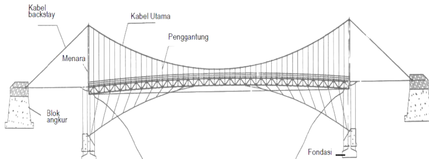
Gambar 1. Skema Jembatan Gantung dan Bagiannya [4]
