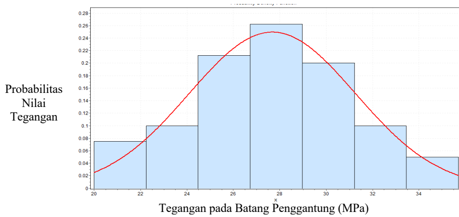
Gambar 9 Distribusi Fungsi Tegangan Batang Penggantung Berbentuk Distribusi Normal (Nilai rata-rata: 27.68 MPa; Standar deviasi: 0.29 MPa)
