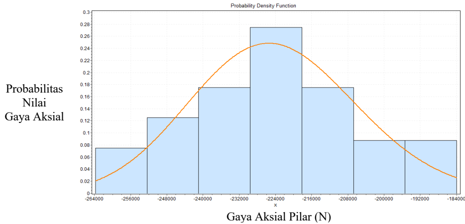
Gambar 11. Distribusi Fungsi Gaya Aksial Pilar Berbentuk Distribusi Log-Normal (Nilai rata-rata: 226.5 kN; Standar deviasi: 0.06 N)
