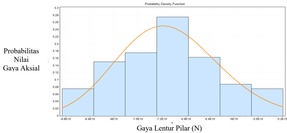
Gambar 12. Distribusi Fungsi Gaya Lentur Pilar Berbentuk Distribusi Log-Normal (Nilai rata-rata: 7.204 kNm; Standar deviasi: 0.09 Nmm)
