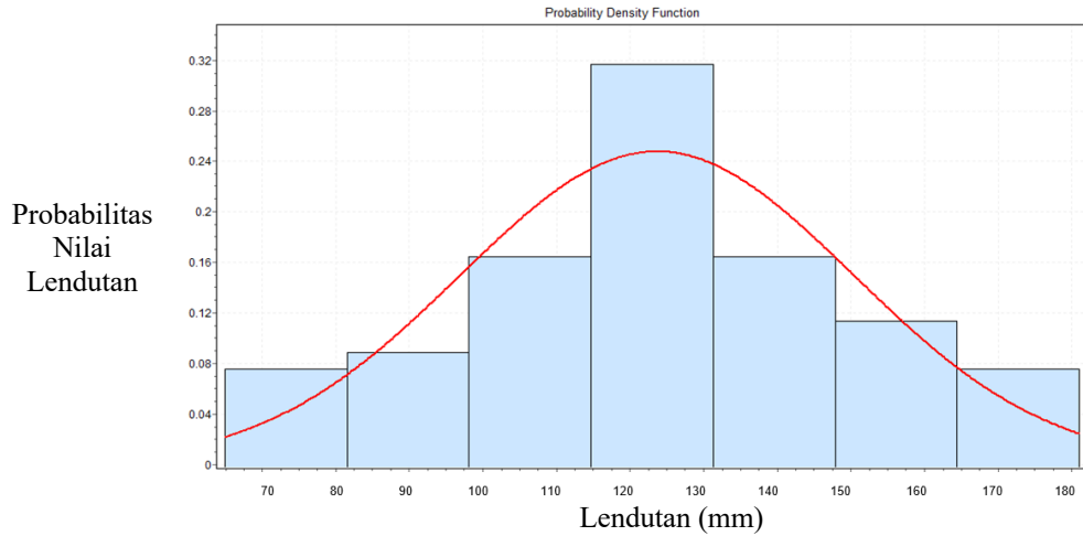
Gambar 8. Distribusi Fungsi Lendutan Berbentuk Distribusi Normal (Nilai rata-rata: 124.54 mm; Standar deviasi: 22.599 mm)
