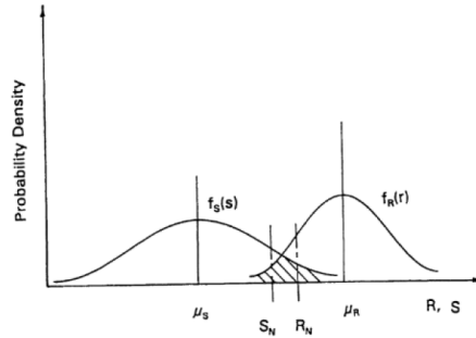
Gambar 2. Probabilitas Kegagalan Struktur
