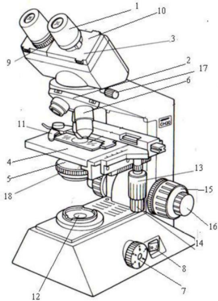
Gambar 1.1. Bagian-bagian Mikroskop (1)
