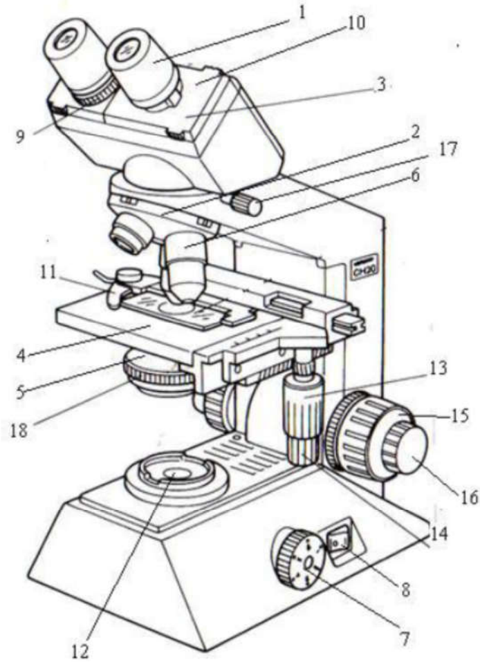
Gambar 1.1. Bagian-bagian Mikroskop 11
