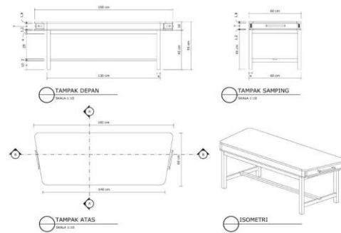
Gambar 1.6 Gambar 3D dan gambar kerja desain meja belajar
