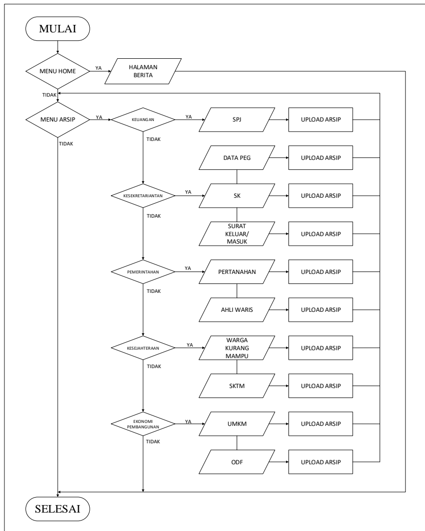
Gambar 1. Flowchart Keseluruhan Sistem Pengelolaan Arsip
