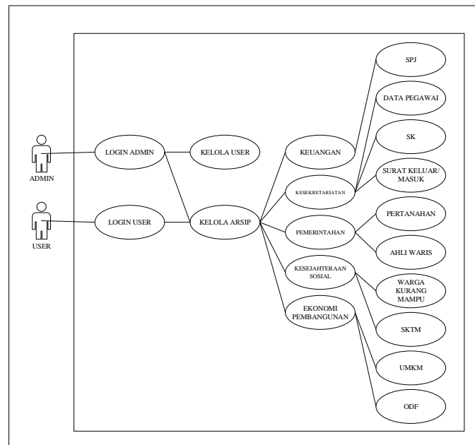
Gambar 2. Use Case Diagram Sistem Pengelolaan Arsip
