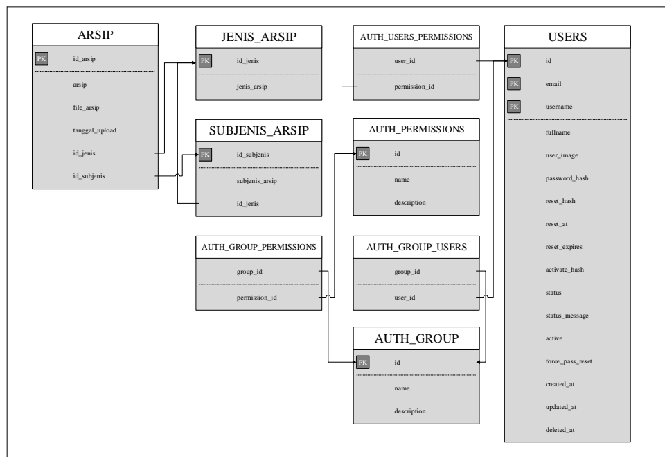
Gambar 3. TRD Sistem Pengelolaan Arsip
