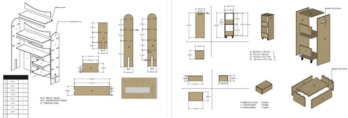
Gambar 15. Gambar Kerja
