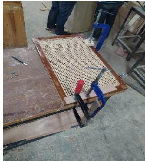
Gambar 13. Proses Perakitan Pintu
