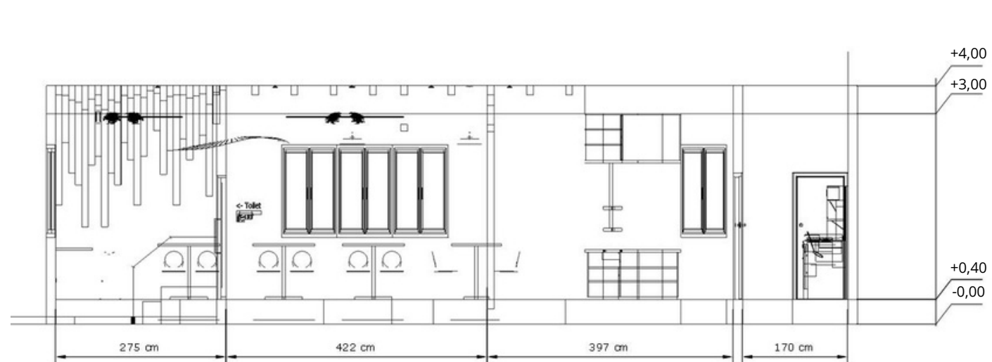
POTONGAN A-A 1:50
