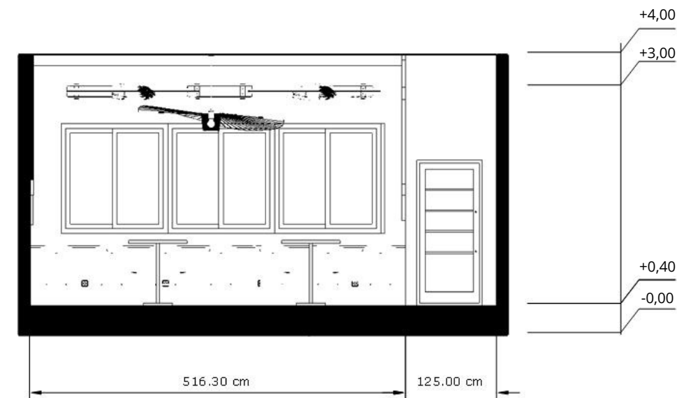
POTONGAN B-B 1:50
