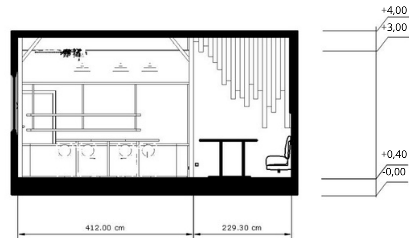
POTONGAN C-C 1:50
