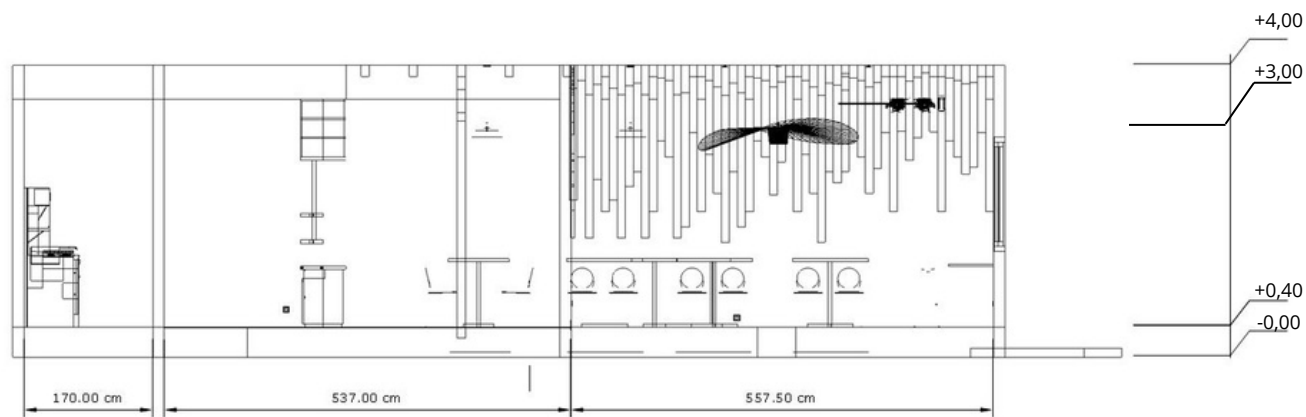
POTONGAN C-C 1:50
