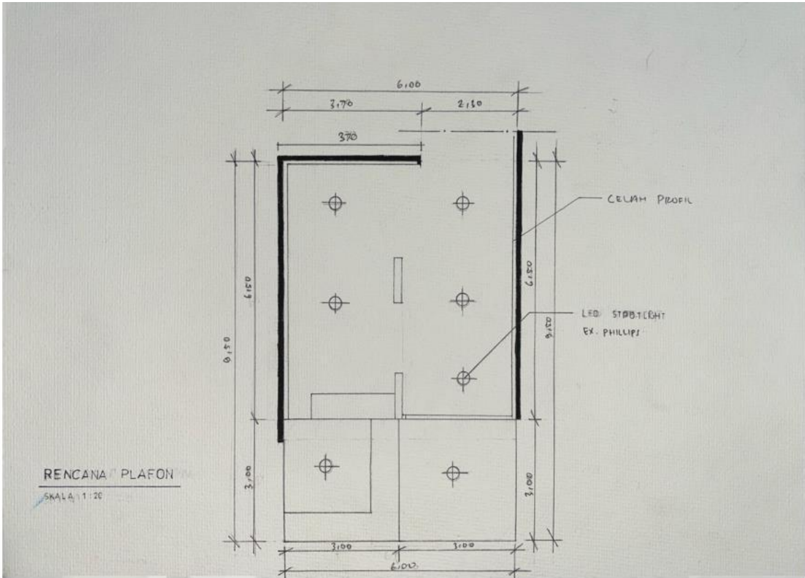
RECANA PLAFON WARUNG 87 RIA RIO
