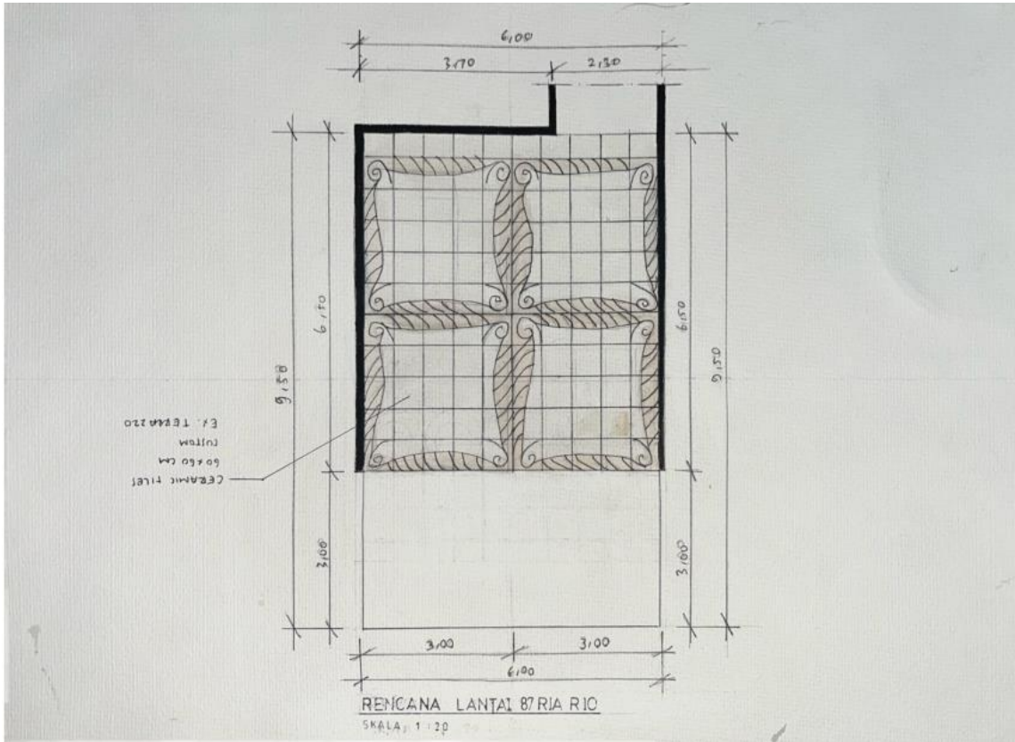
RENCANA LANTAI WARUNG 87 RIA RIO
