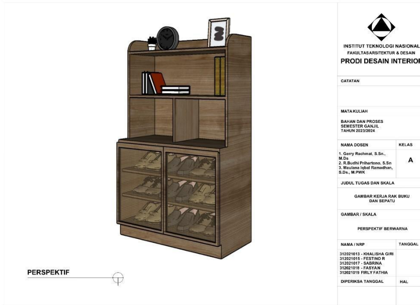
Gambar 22. Gambar Kerja Prototype
