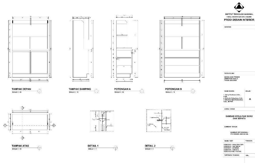
Gambar 20. Gambar Kerja Prototype
