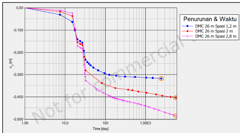
Gambar 11. Grafik perbandingan hasil pemodelan variasi jarak DMC
