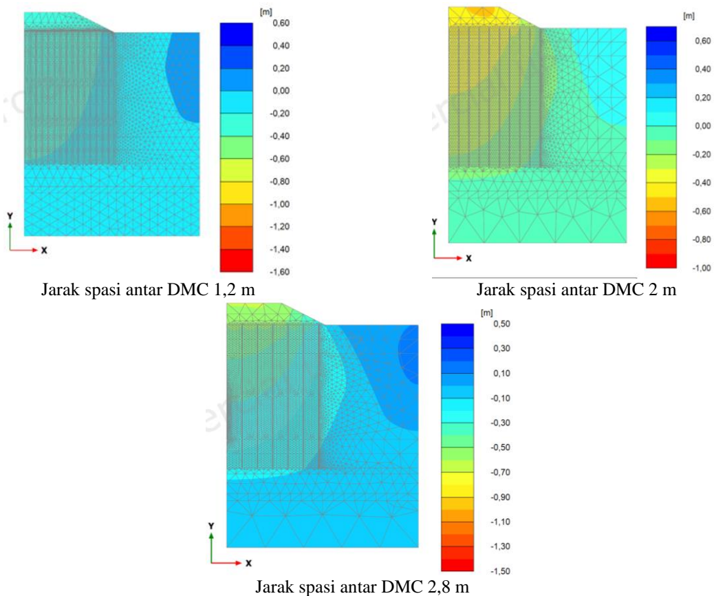
Gambar 10. Deformasi perbaikan tanah dengan metode preloading kombinasi variasi jarak DMC
