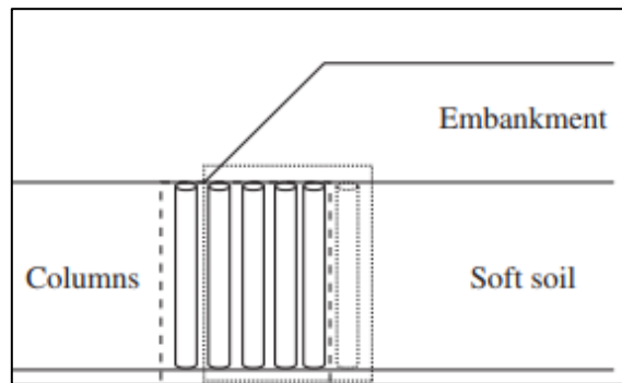
Gambar 4. Skema perbaikan dengan Deep Mixing Column (Han, 2015)
