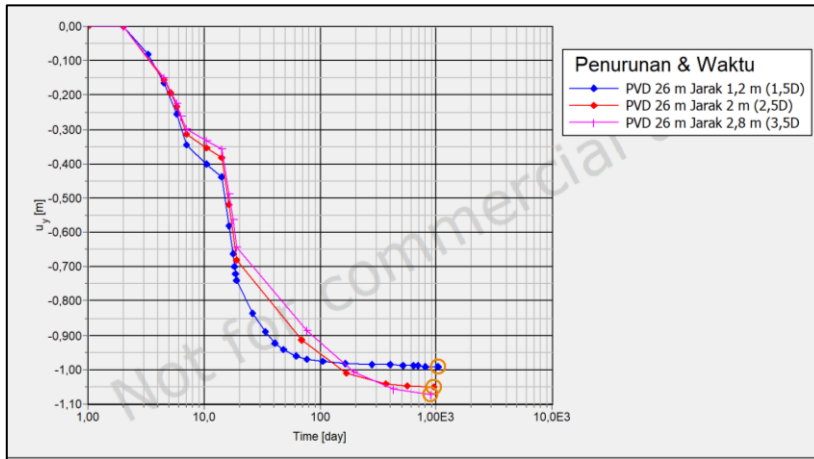
Gambar 7. Grafik perbandingan hasil pemodelan variasi jarak PVD
