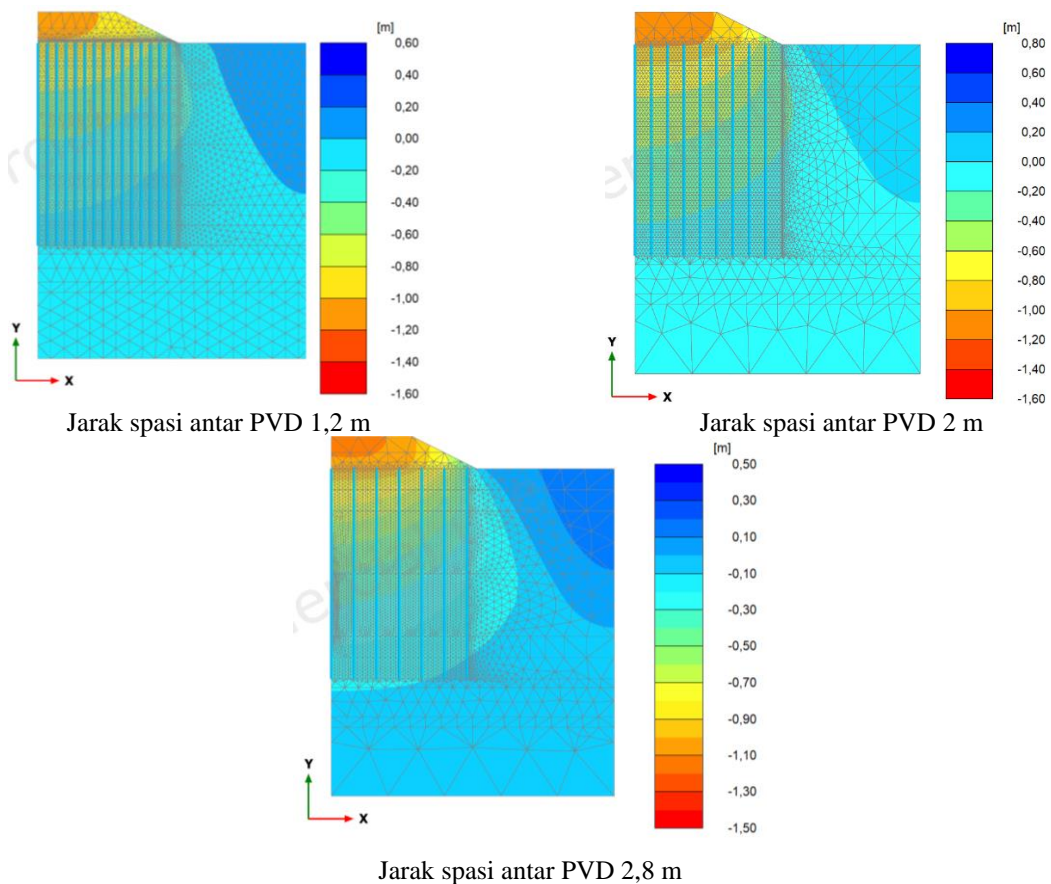
Gambar 6. Deformasi perbaikan tanah dengan metode preloading kombinasi variasi jarak PVD
