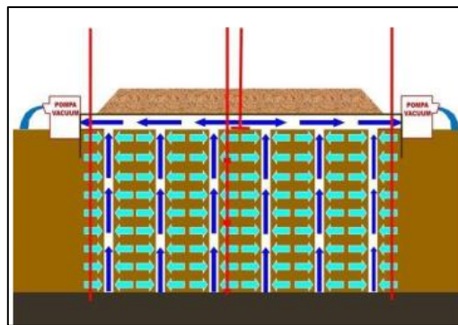
Gambar 2. Skema perbaikan tanah dengan vacuum preloading (Kuswanda, 2016)
