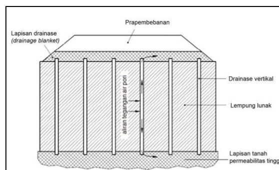
Gambar 3. Skema perbaikan dengan prefabricated vertical drain (Badan Standarisasi Nasional, 2017)
