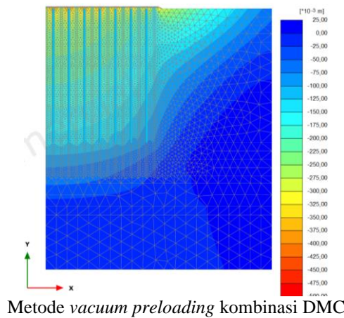
Gambar 14 (lanjutan). Deformasi tanah dengan beberapa metode perbaikan tanah
