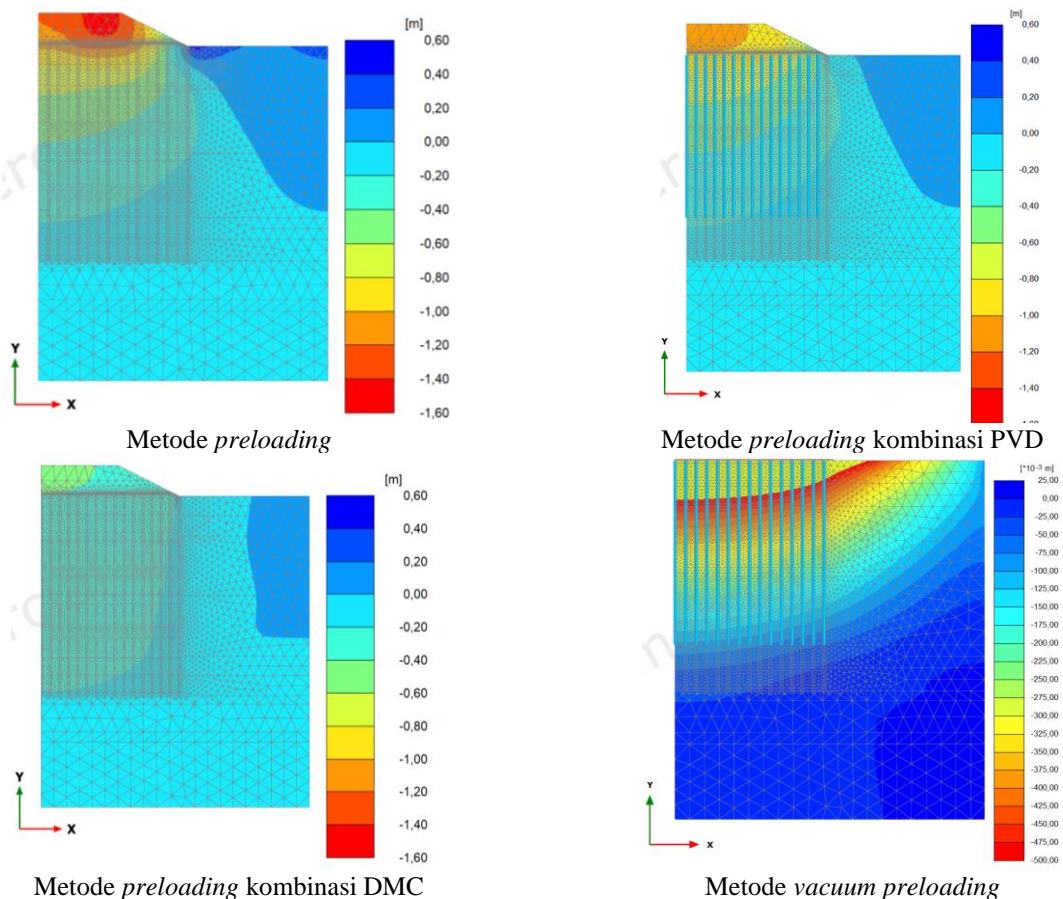
Gambar 14. Deformasi tanah dengan beberapa metode perbaikan tanah
