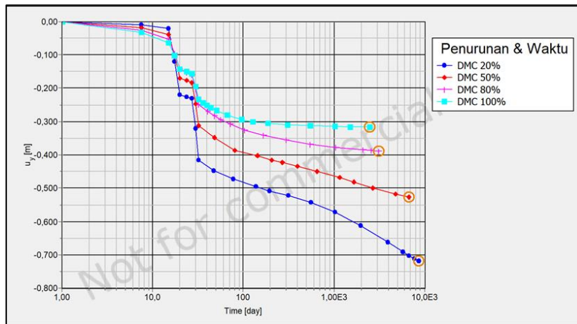
Gambar 13. Grafik perbandingan hasil pemodelan variasi kedalaman DMC
