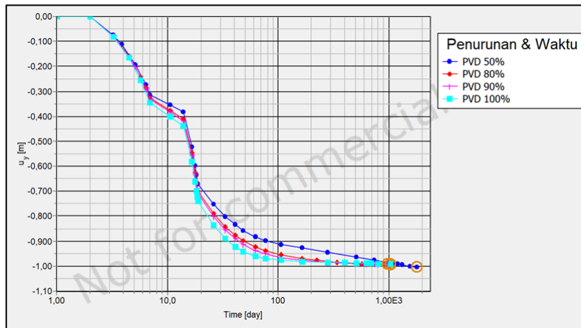
Gambar 9. Grafik perbandingan hasil pemodelan variasi kedalaman PVD
