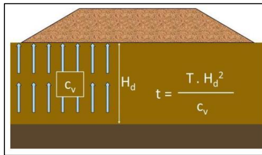
Gambar 1. Skema perbaikan tanah dengan preloading (Kuswanda, 2016)
