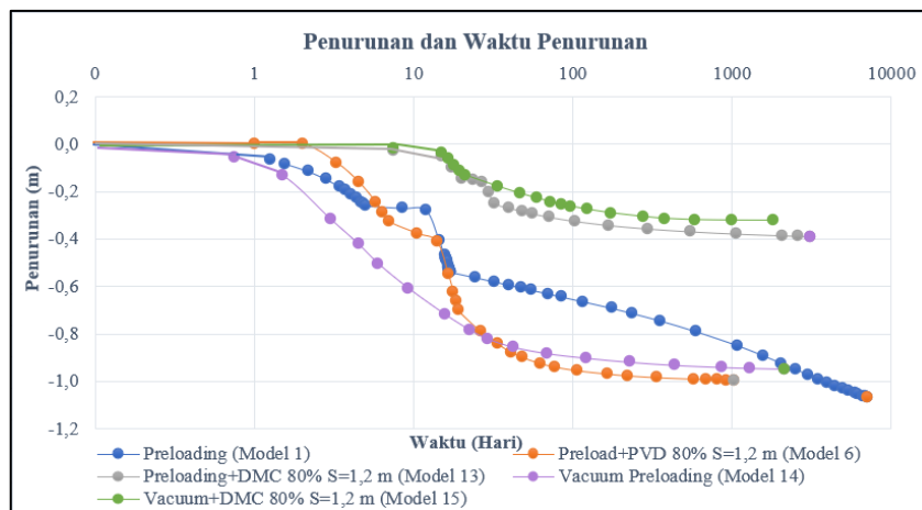
Gambar 15. Grafik perbandingan hasil pemodelan dengan berbagai macam metode perbaikan tanah
