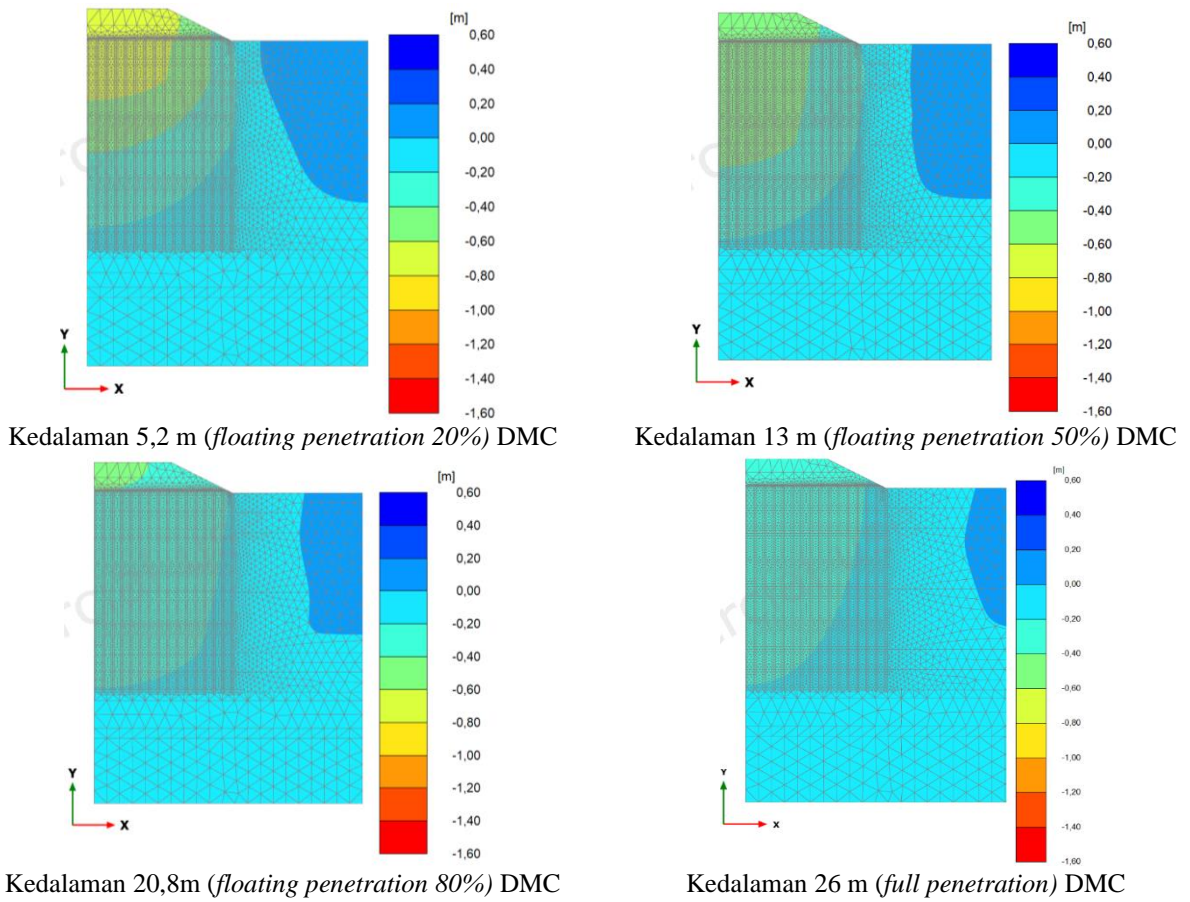
Gambar 12. Deformasi perbaikan tanah dengan metode preloading kombinasi variasi kedalaman DMC
