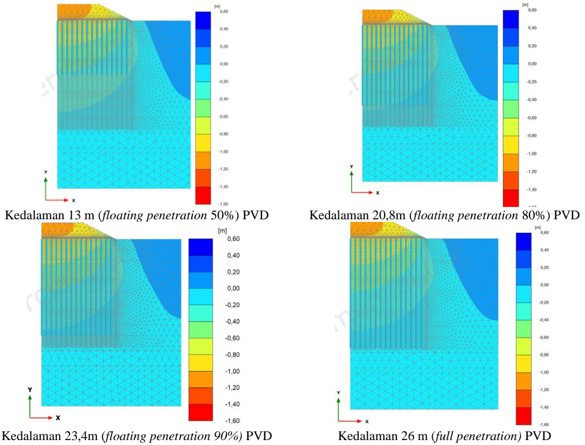
Gambar 8. Deformasi perbaikan tanah dengan metode preloading kombinasi variasi kedalaman PVD
