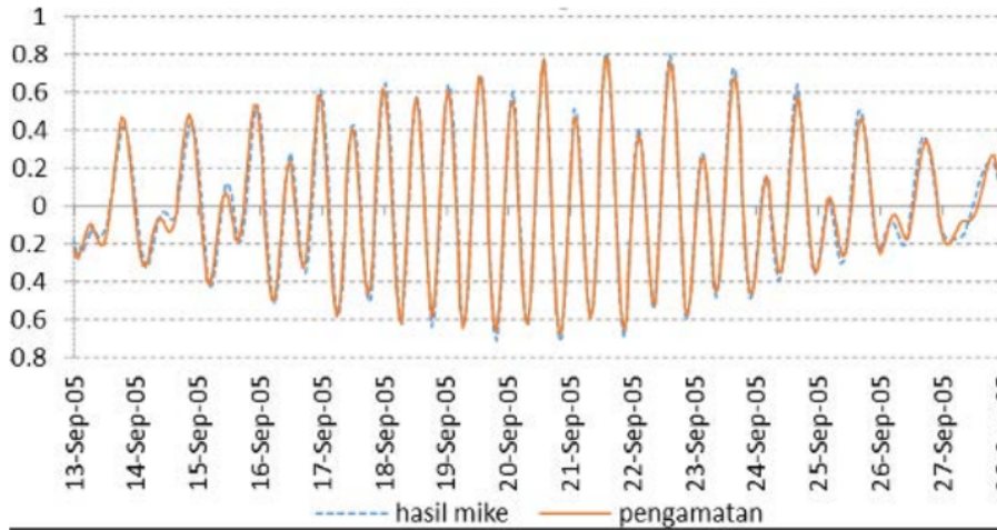
Gambar 2. Validasi elevasi muka air
