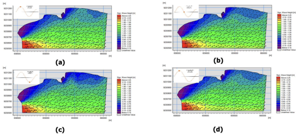
Gambar 6. Hasil Pemodelan Existing Musim Barat
