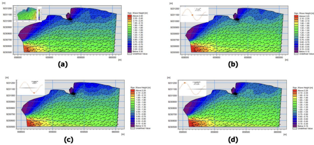
Gambar 9. Hasil Pemodelan Alternatif 1 Musim Barat
