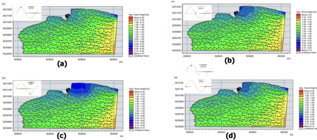
Gambar 5. Hasil Pemodelan Existing Musim Timur
