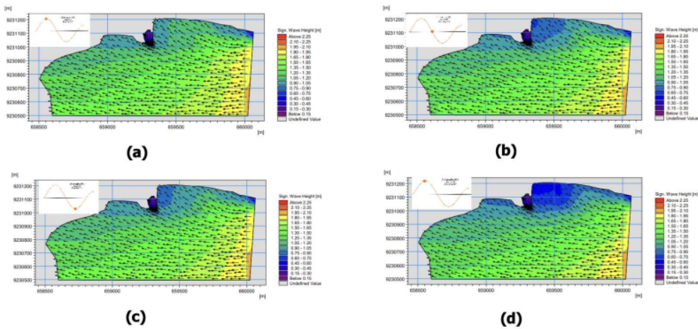
Gambar 8. Hasil Pemodelan Alternatif 1 Musim Timur
