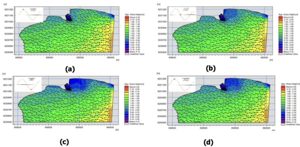
Gambar 11. Hasil Pemodelan Alternatif 2 Musim Timur
