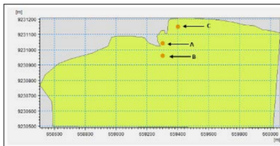
Gambar 4. Titik Lokasi Kondisi Existing (sumber: MIKE 21 SW)
