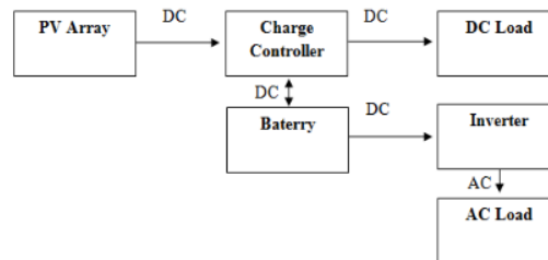
Gambar 4. Skema sistem off grid [16]
