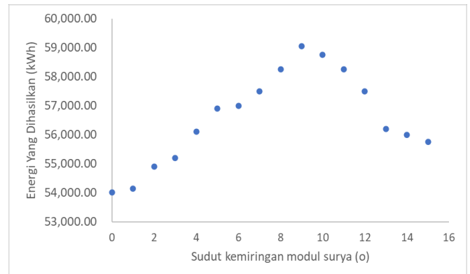
Gambar 13. Energi Yang Dihasilkan Terhadap Sudut Kemiringan Modul Surya
