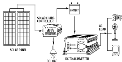
Gambar 5. Skema peralatan PLTS off grid [16]
