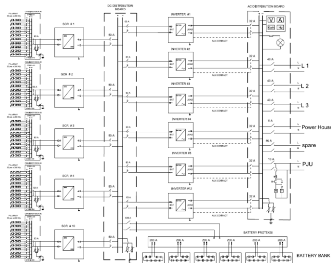
Gambar 15. Wiring diagram sistem PLTS hasil perancangan
