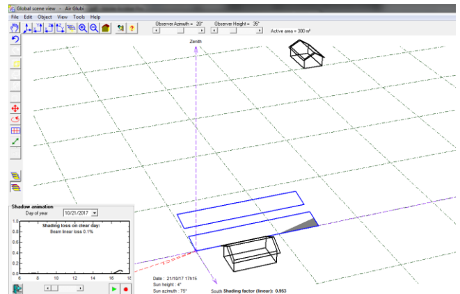
Gambar 9. Hasil simulasi shading PLTS Air Glubi pada jam 17.00
