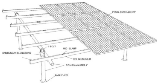
Gambar 14. Struktur penyangga modul surya hasil perancangan
