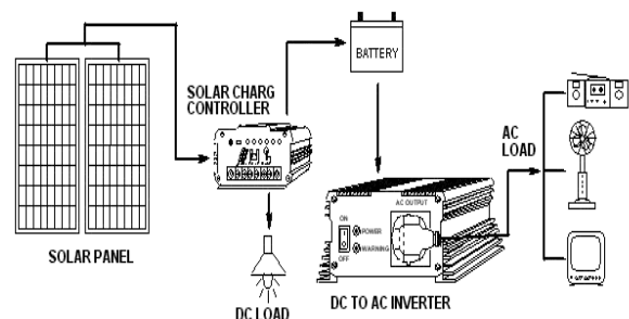
Gambar 5. Skema peralatan PLTS off grid [16]
