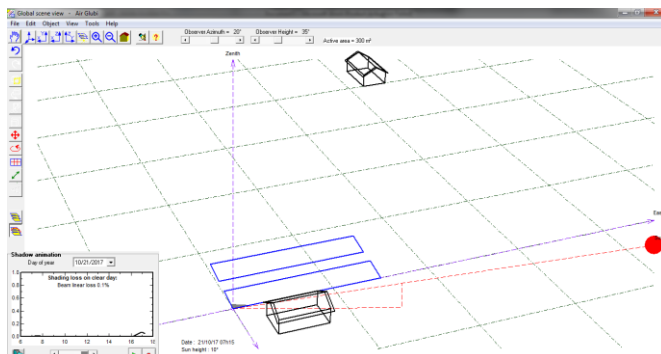
Gambar 11. Hasil simulasi shading PLTS Air Glubi pada jam 7.00
