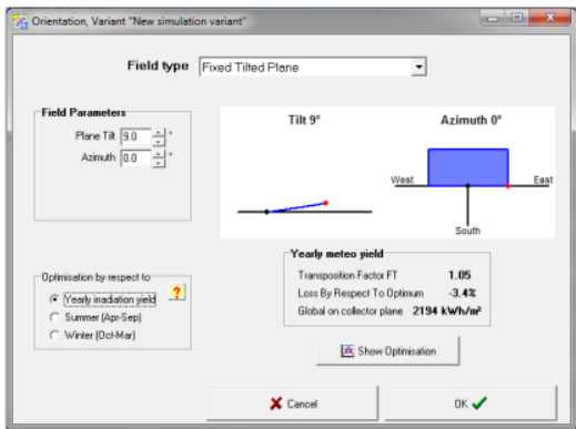
Gambar 7. Optimasi kemiringan modul surya
