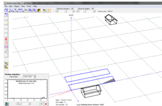
Gambar 9. Hasil simulasi shading PLTS Air Glubi pada jam 17.00
