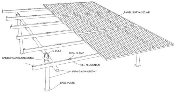
Gambar 14. Struktur penyangga modul surya hasil perancangan
