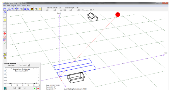
Gambar 10. Hasil simulasi shading PLTS Air Glubi pada jam 12.00
