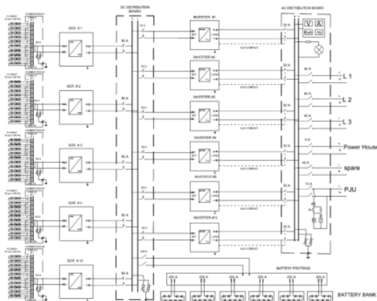
Gambar 15. Wiring diagram sistem PLTS hasil perancangan
