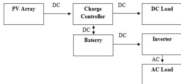
Gambar 4. Skema sistem off grid [16]
