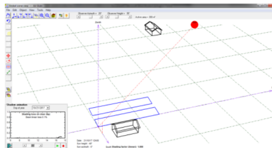
Gambar 10. Hasil simulasi shading PLTS Air Glubi pada jam 12.00
