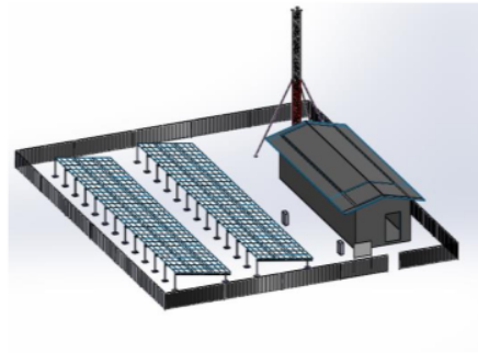
Gambar 8. Optimasi layout PLTS
