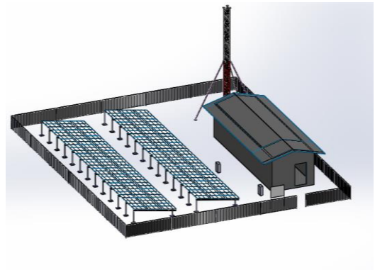
Gambar 8. Optimasi layout PLTS
