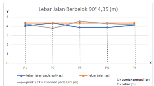
Gambar 16 Grafik lebar jalan berkelok 90°
