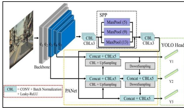
Gambar 2. Struktur YOLOv4
