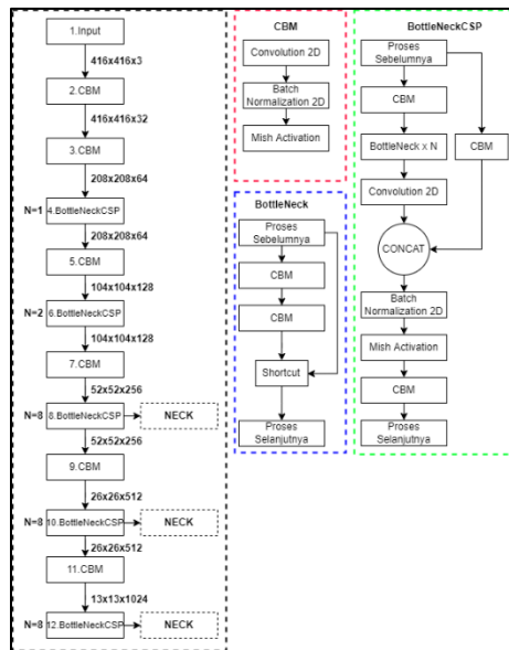
Gambar 3. Struktur CSPDarknet53
