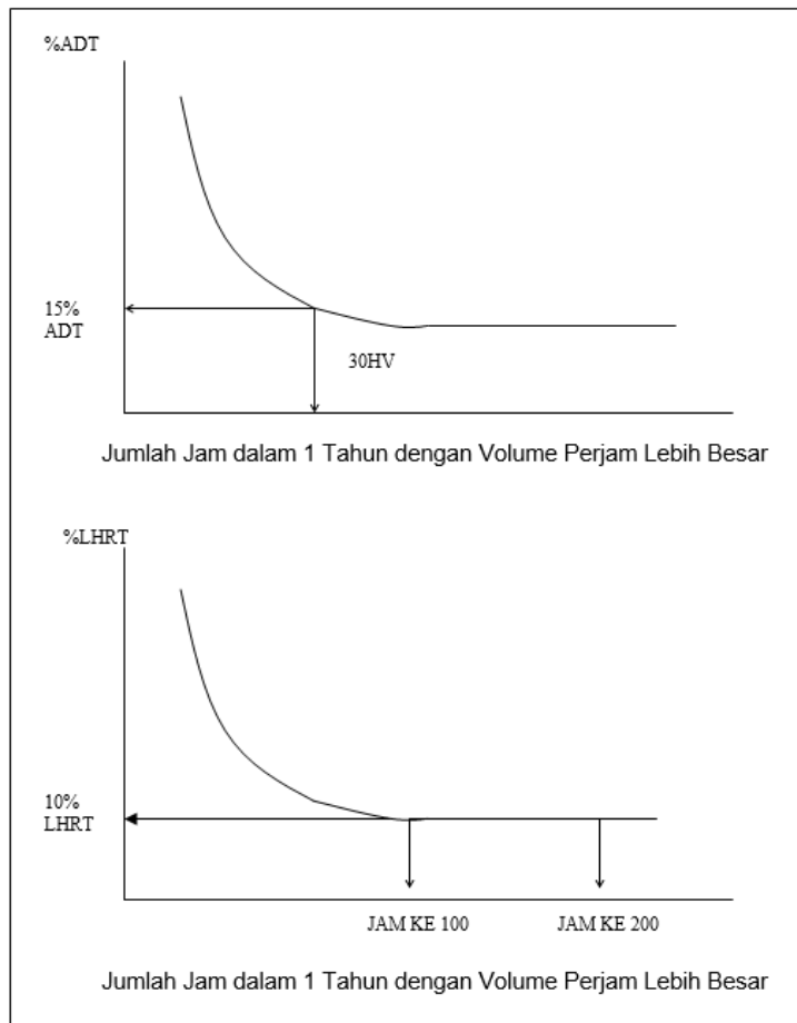
Gambar 2.2 Penentuan Volume Jam Perencanaan
