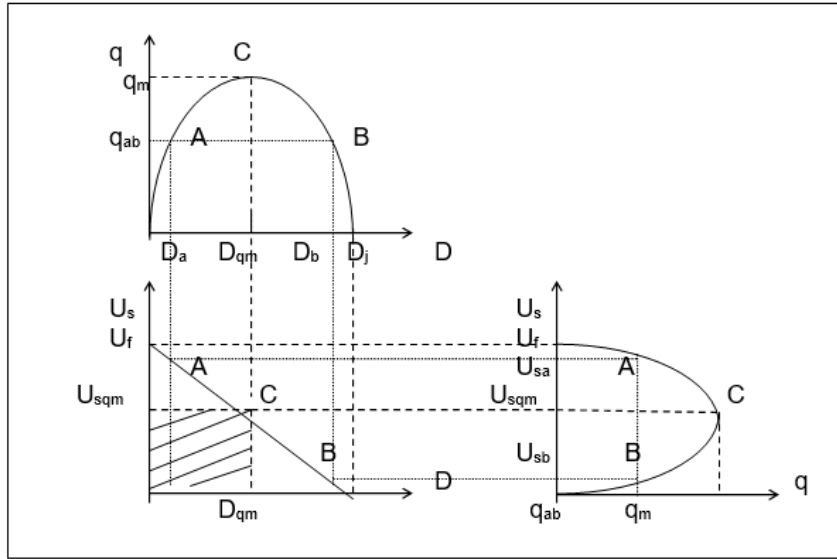
Gambar 3.2 Hubungan antara Arus-Kecepatan Rata-Rata Ruang dan Kerapatan
