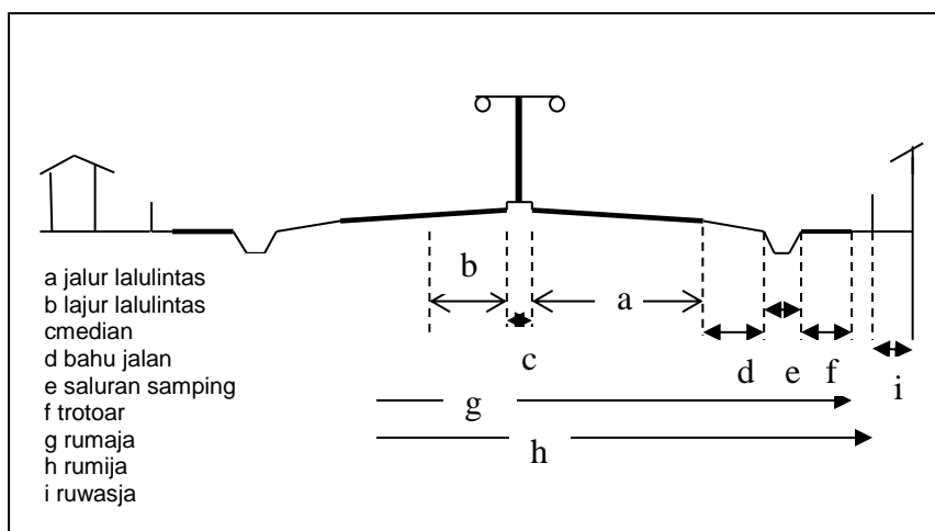
Gambar 1.3 Tipikal Potongan Melintang Jalan
