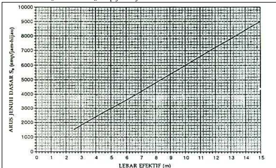
Gambar . Arus Jenuh Dasar Untuk Pendekat Tipe P
