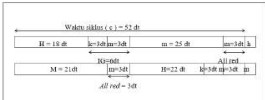
Gambar 7.6 Diagram Waktu
