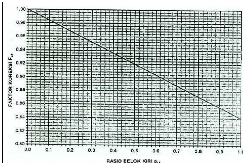
Gambar Faktor Penyesuaian Belok Kiri ( F_{LT} )
