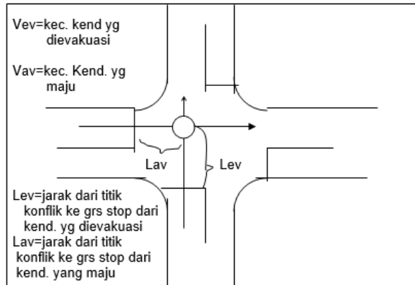
Gambar 6.5. Penentuan titik Konflik Kritis
