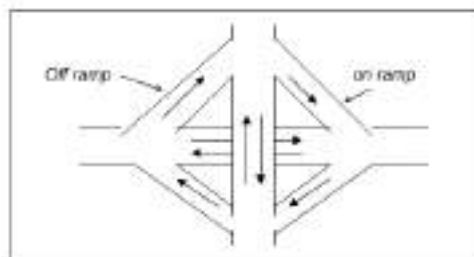
Gambar 5.2 Persimpangan Tidak Sebidang
