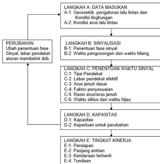
Gambar 6.5. Bagan Alir untuk Analisis APILL
