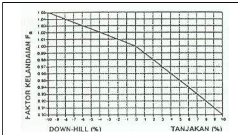
Gambar . Faktor Penyesuaian Untuk Kelandaian ( F_G )
