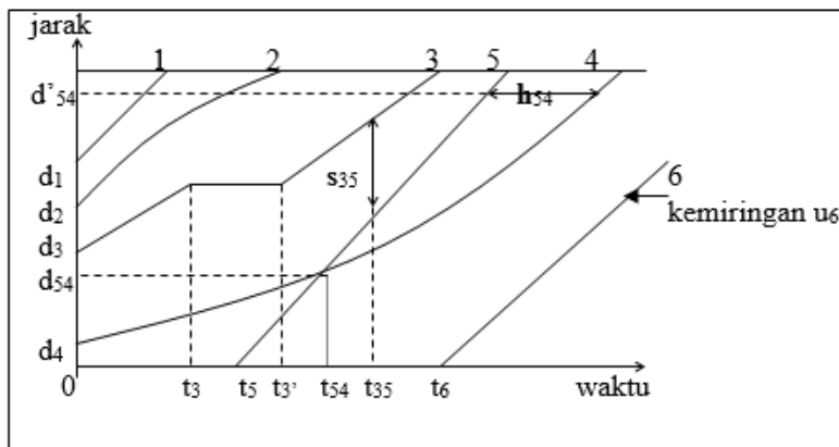
Gambar 3.1 Diagram Ruang dan Waktu
