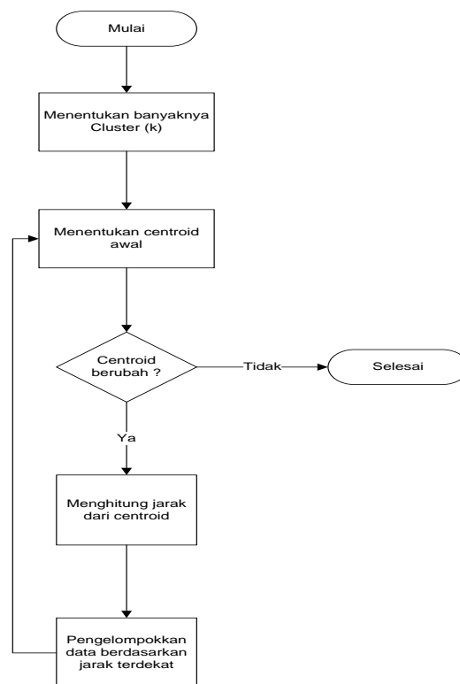
Gambar 1. Algoritma K-means
