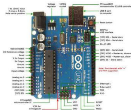
Figure 6. Arduino Uno
