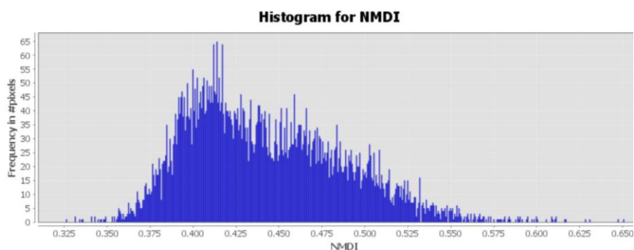
Gambar 5. Grafik Kekeringan Indeks Vegetasi NMDI
