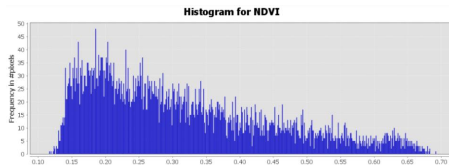
Gambar 7. Grafik Kekeringan Indeks Vegetasi NDVI
