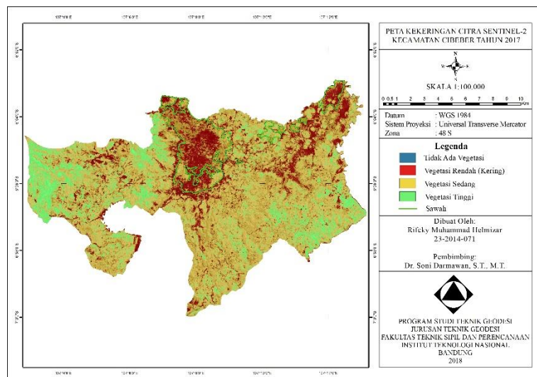
Gambar 6. Hasil Peta Kekeringan Berdasarkan Indeks NDVI
