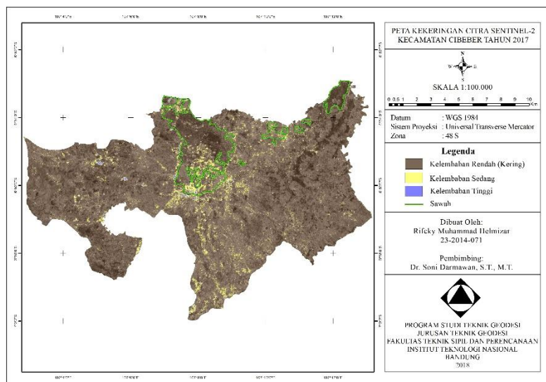
Gambar 4. Hasil Peta Kekeringan Berdasarkan Indeks NMDI
