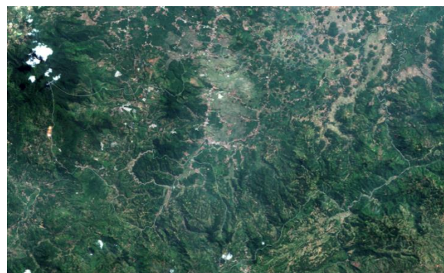
Gambar 3. RGB 432 Citra Sentinel-2 Kecamatan Cibeber
