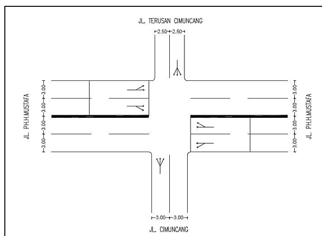
Gambar 2. Geometri persimpangan
