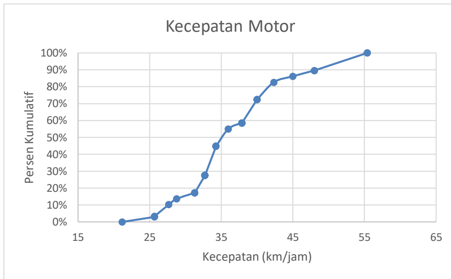
Gambar 5. Grafik distribusi kecepatan motor
