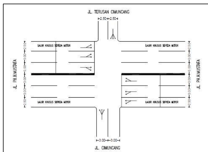
Gambar 7. Skenario pemodelan desain
