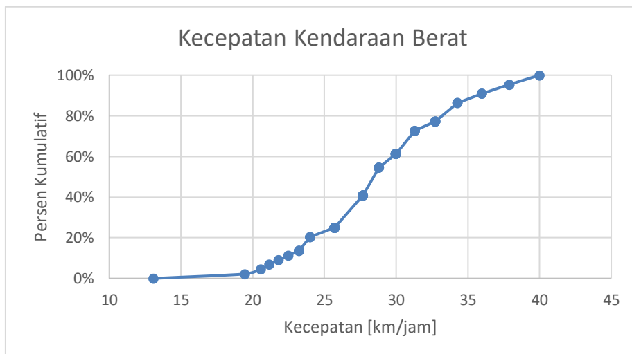
Gambar 6. Grafik distribusi kecepatan kendaraan berat
