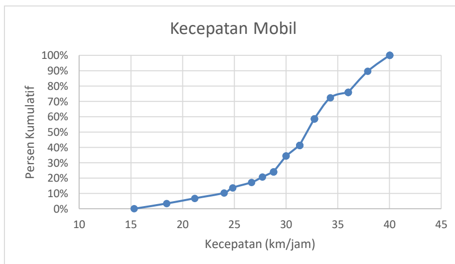
Gambar 4. Grafik distribusi kecepatan mobil
