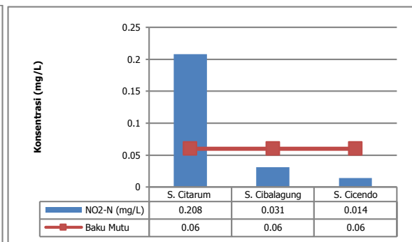
Gambar 3. Konsentrasi Nitrit
