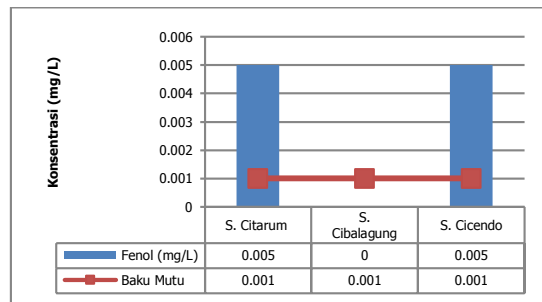
Gambar 6. Konsentrasi Fenol
