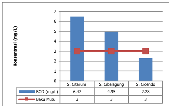
Gambar 2. Konsentrasi BOD
